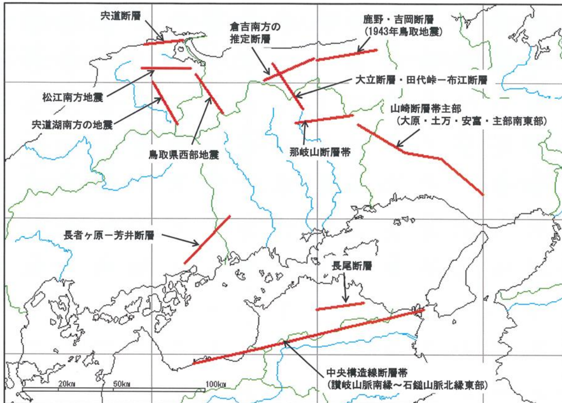
各断層の位置 (資料：岡山県地域防災計画)
